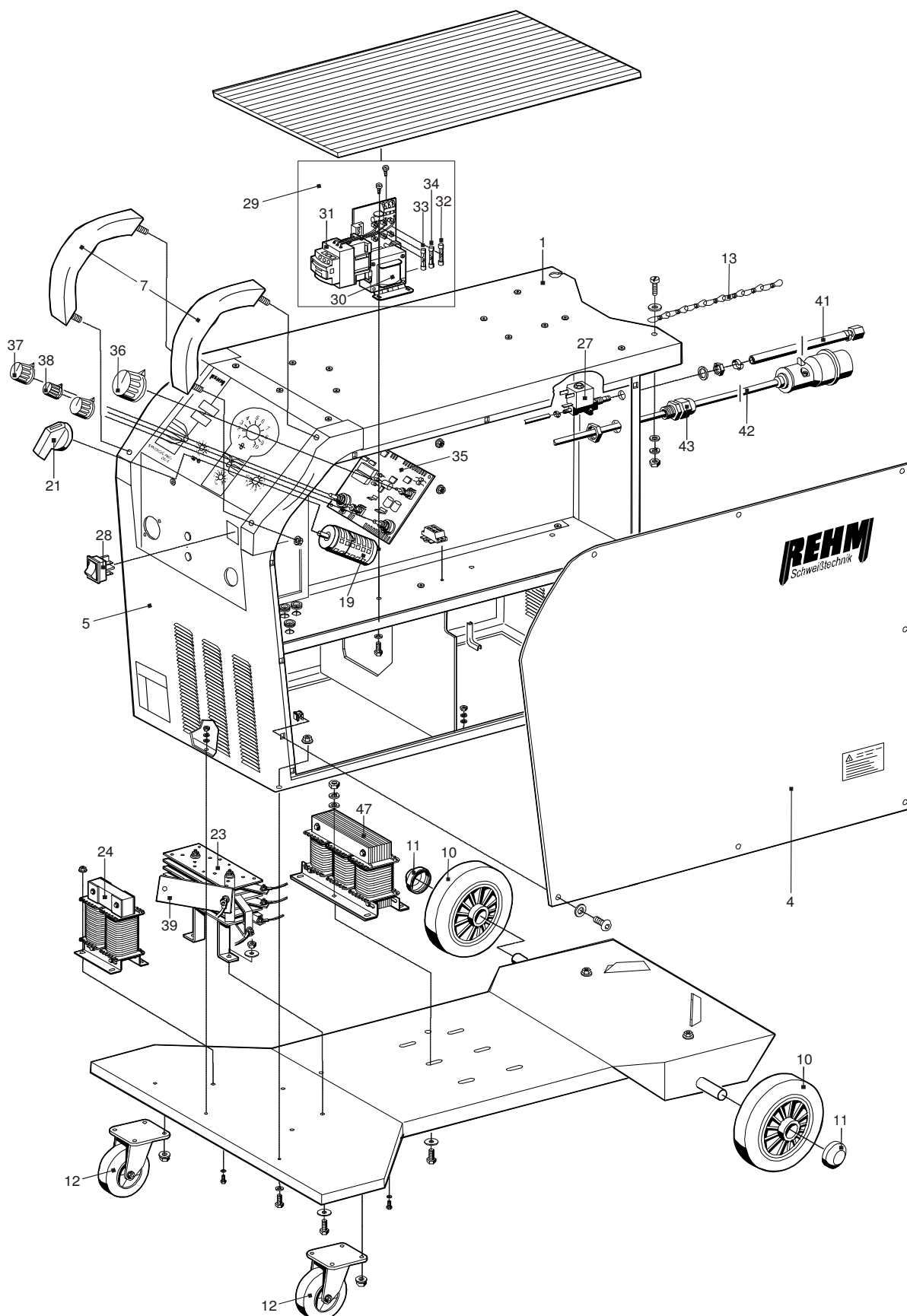
Abb.5: Explosionszeichnung SYNERGIC.PRO² 250-4 – 450-4W
